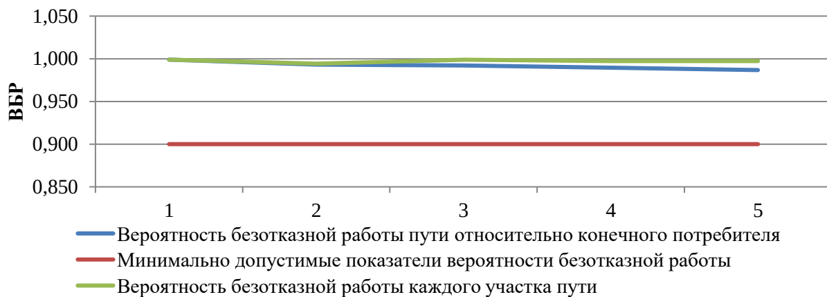
Рисунок 51. ВБР относительно участка тепловой сети от камеры «Вывод - Котельная № 31» до потребителя «Школа № 1, мастерские»
