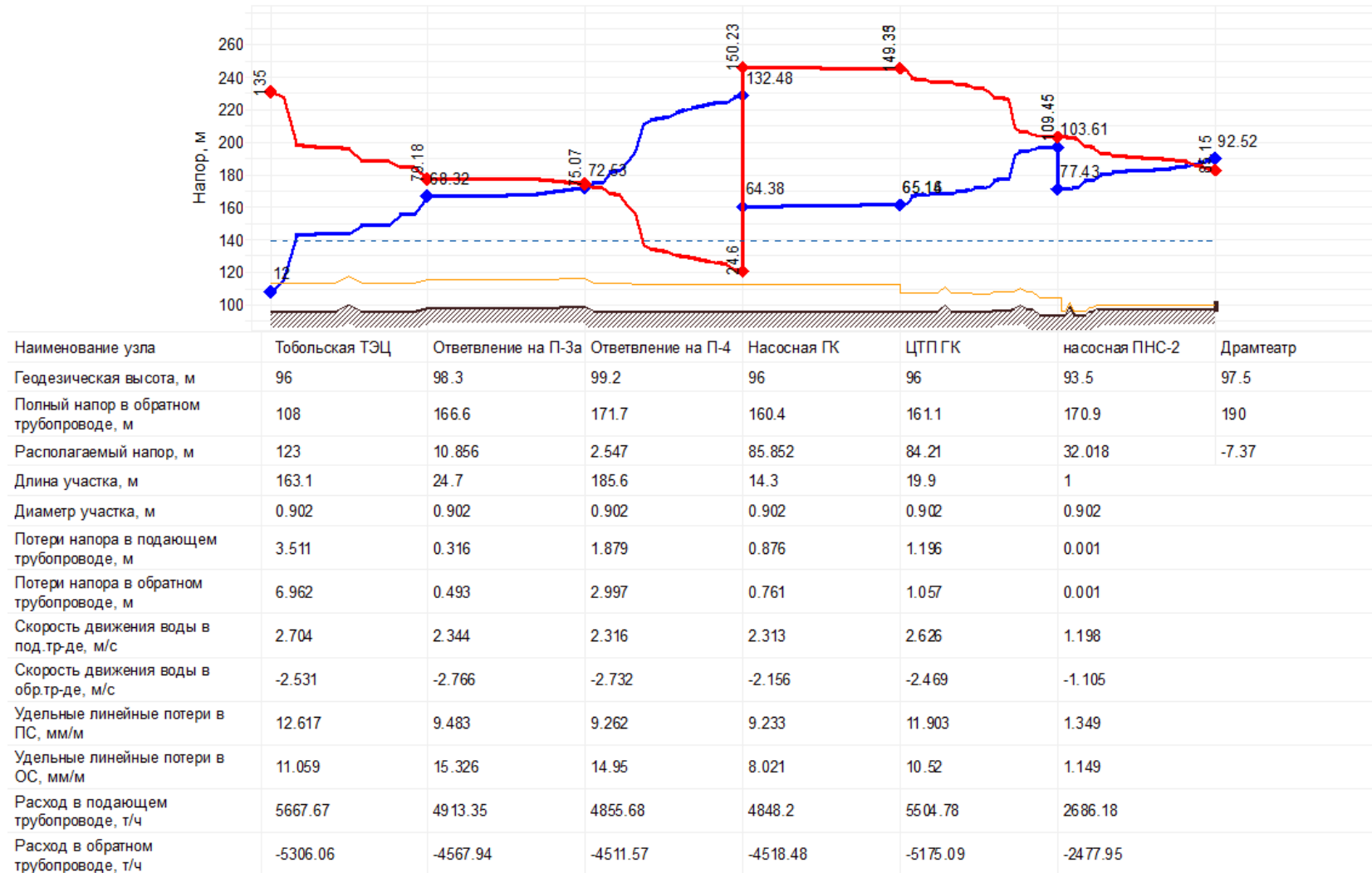
Рисунок 18. Пьезометрический график тепловой сети от ЭТПГ до потребителя «Драмтеатр»
