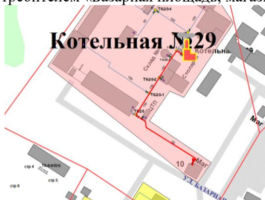
Рисунок 48. Трассировка участка тепловой сети от камеры «Вывод - Котельная № 29» до потребителя «Базарная площадь, магазин»
