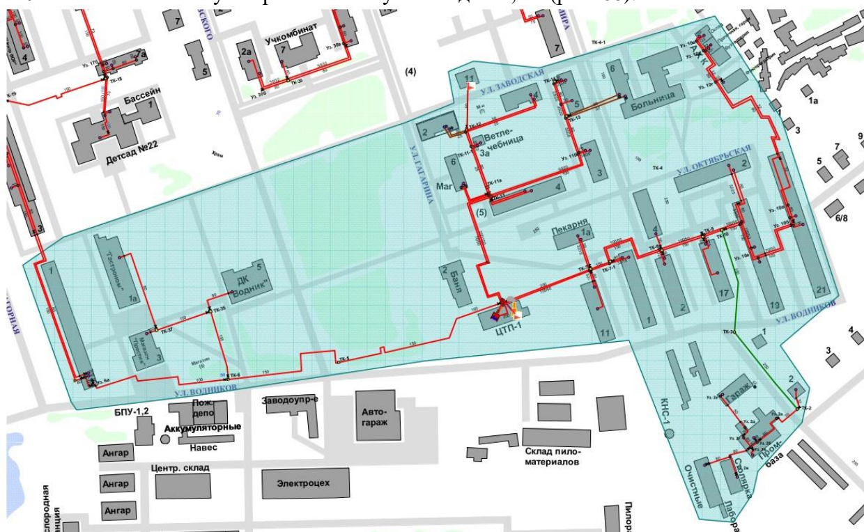
Рисунок 68. Трассировка участка тепловой сети от камеры «Вывод - Котельная № 9» до потребителя по ул. Заводская, 11
