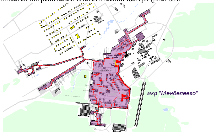
Рисунок 60. Трассировка участка тепловой сети от камеры «Вывод - Котельная № 22» до потребителя «Эстетический центр»
