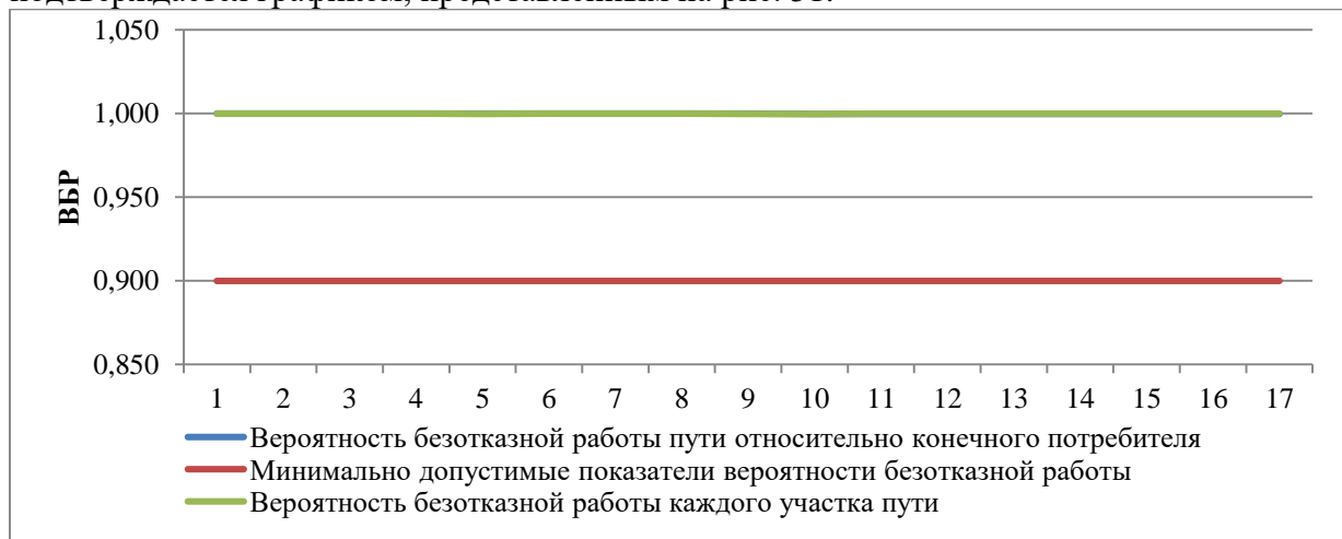
Рисунок 51. ВБР относительно участка тепловой сети от камеры «Вывод - Котельная № 27» до потребителя ул. Лермонтова, 7, АБК
