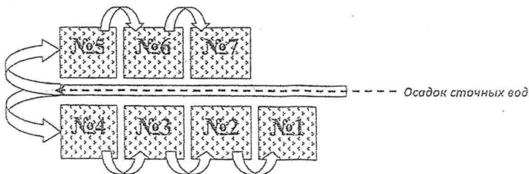
Рисунок 12. Схема расположения иловых карт
