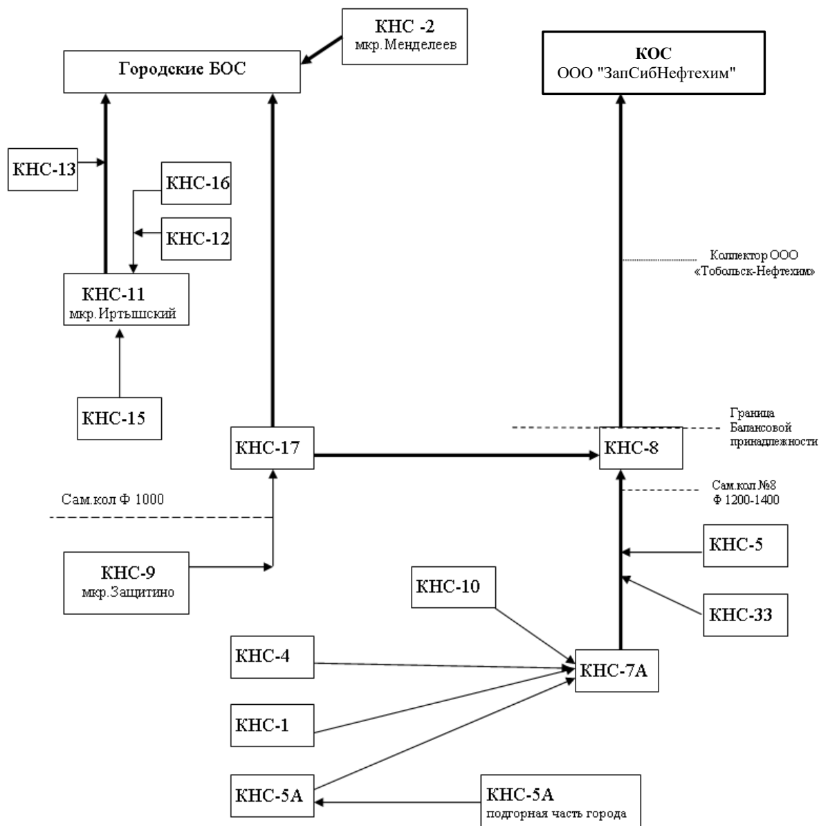
Рисунки 6. Организационная схема перекачки стоков города Тобольска
