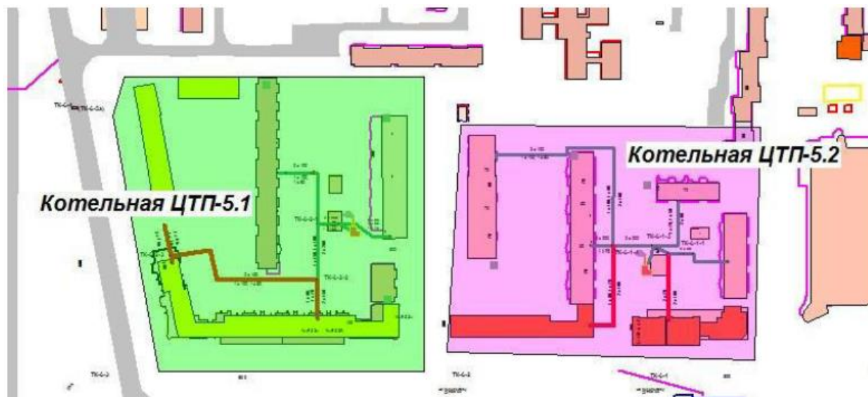
Рисунок 15. Перспективная схема зон действия централизованной системы горячего водоснабжения с привязкой к топографической основе города Тобольска (7а мкр., ЦТП-Тобольск-Полимер)
