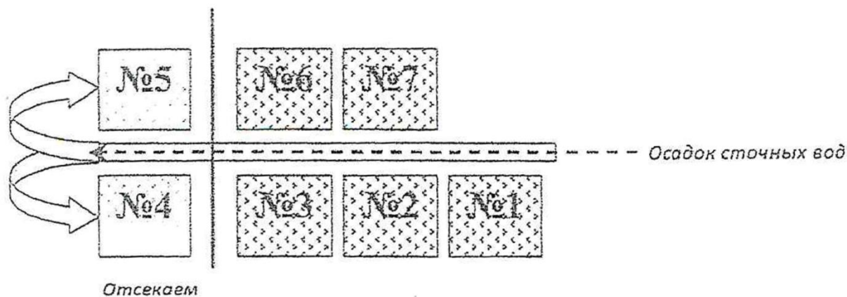
Рисунок 13. Схема очистки иловых карт
