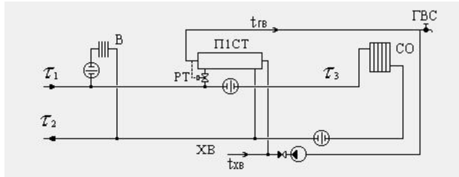
Рисунок 5. Схема технологического присоединения потребителей мкр. Иртышский
