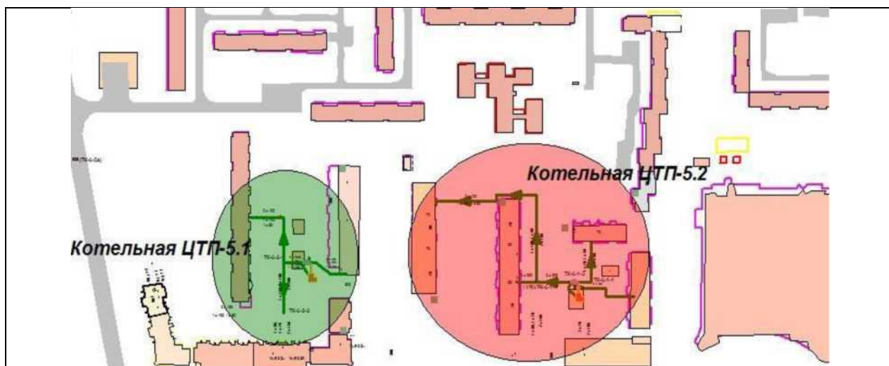
Рисунок 3. Графическое отображение зон действия централизованной системы горячего водоснабжения с привязкой к топографической основе города Тобольска (7 мкр., ЦТП-5.1, 5.2)
