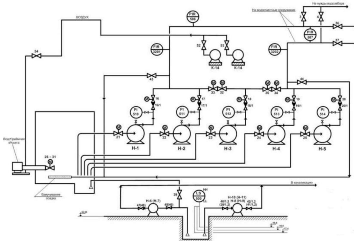
Рисунок 3. Технологическая схема Епанчинского водозабора.
