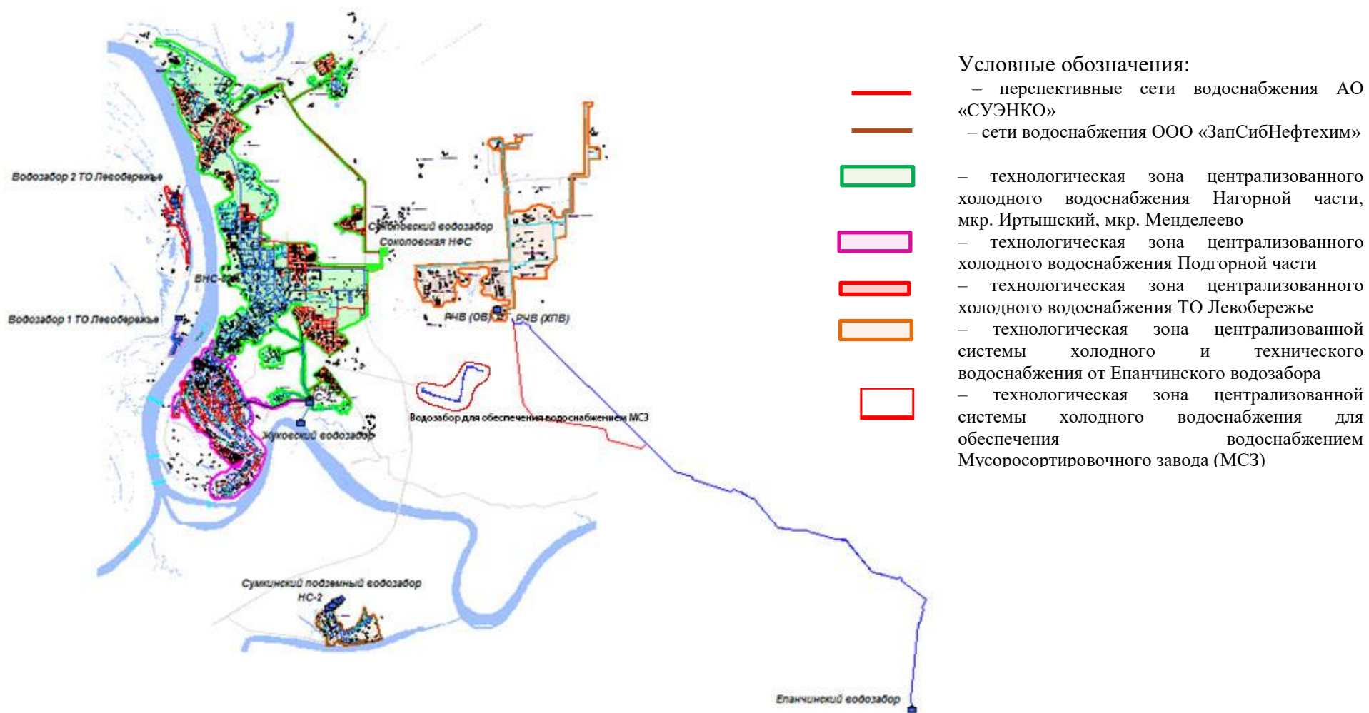
Рисунок 1. Зоны с централизованными системами водоснабжения города Тобольска на перспективу до 2032 года (с выделением технологических зон водоснабжения)
