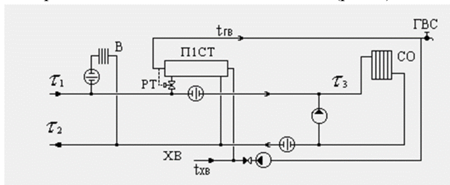
Рисунок 4. Схема технологического присоединения потребителей к ЦТП
