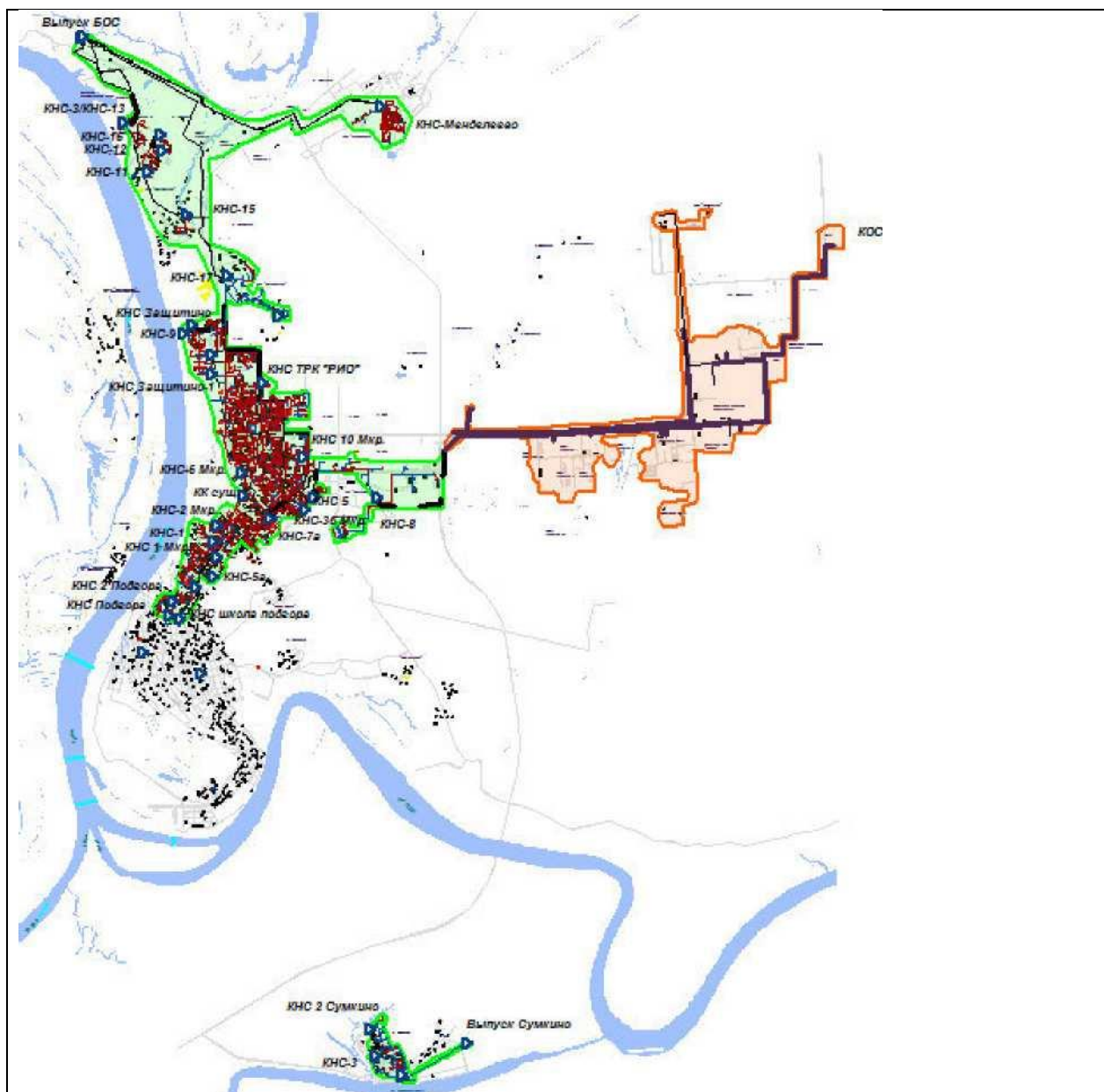
Рисунок 2. Графическое отображение объектов централизованной системы водоотведения с привязкой к топографической основе города Тобольска
