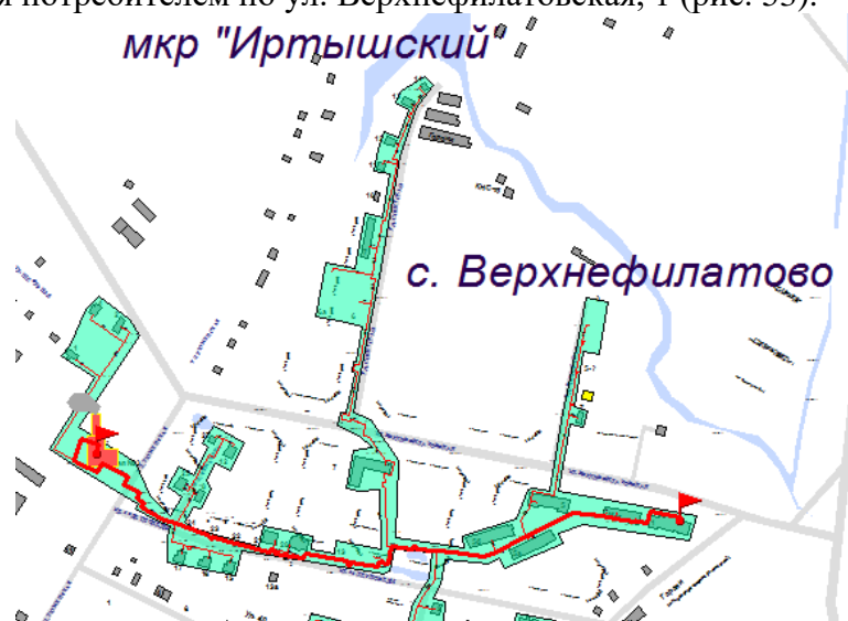
Рисунок 53. Трассировка участка тепловой сети от камеры вывод Котельная № 3 до потребителя по ул. Верхнефилатовская, 1
