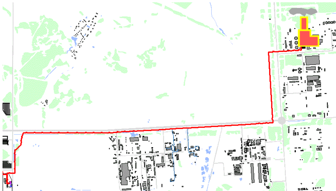
Рисунок 23. Трассировка тепловой сети от Тобольской ТЭЦ до ГК-1
