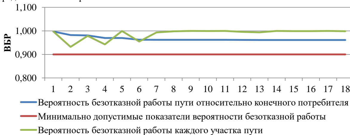
Рисунок 68. ВБР относительно участка тепловой сети от камеры «Вывод - Котельная № 11» до потребителя по ул. Водников, 3.
