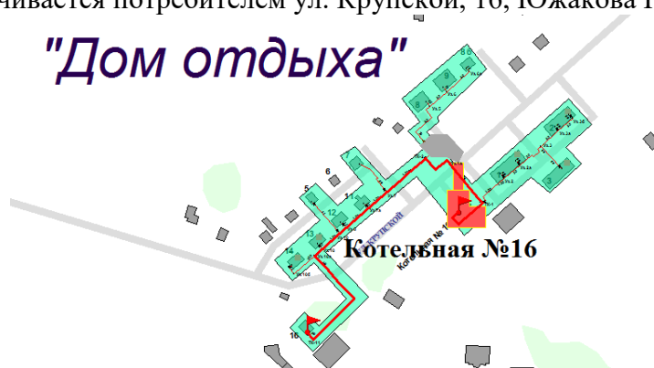
Рисунок 59. Трассировка участка тепловой сети от камеры «Вывод - Котельная № 16» до потребителя ул. Крупской, 16, Южакова Г.Г.
