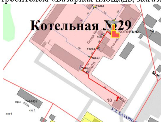
Рисунок 49. Трассировка участка тепловой сети от камеры «Вывод - Котельная № 29» до потребителя «Базарная площадь, магазин»
