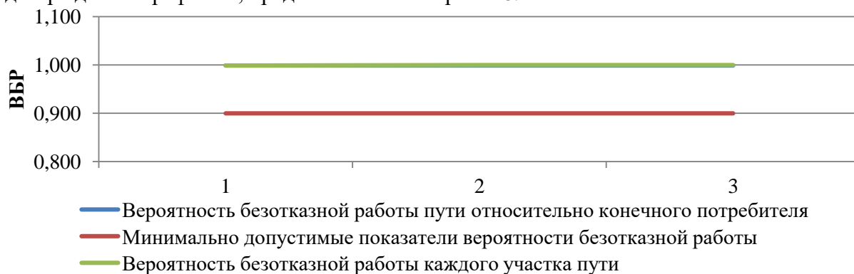
Рисунок 46. ВБР относительно участка тепловой сети от камеры «Вывод - Котельная № 24» до потребителя «Детский сад № 5 «Голубок»
