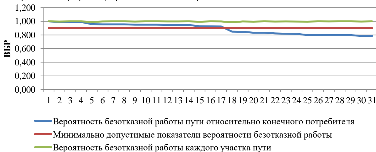
Рисунок 54. ВБР относительно участка тепловой сети от камеры «Вывод - Котельная № 3» до потребителя по ул. Верхнефилатовская, 1
