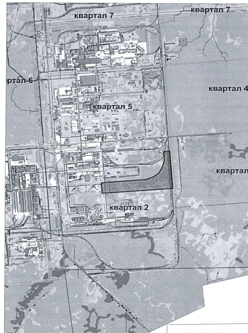
Ситуационный план территории с указанием границ проектирования
