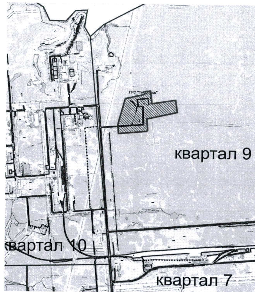
Ситуационный план территории с указанием границ проектирования
