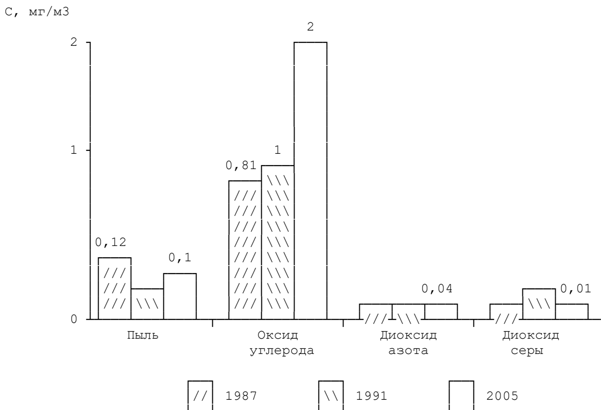
Фоновые концентрации загрязняющих веществ в атмосферном воздухе
