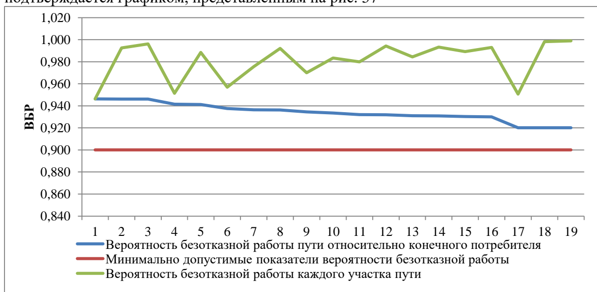
Рисунок 57. ВБР относительно участка тепловой сети от камеры «Вывод - Котельная № 16» до потребителя ул. Крупской, 16, Южакова Г.Г.
