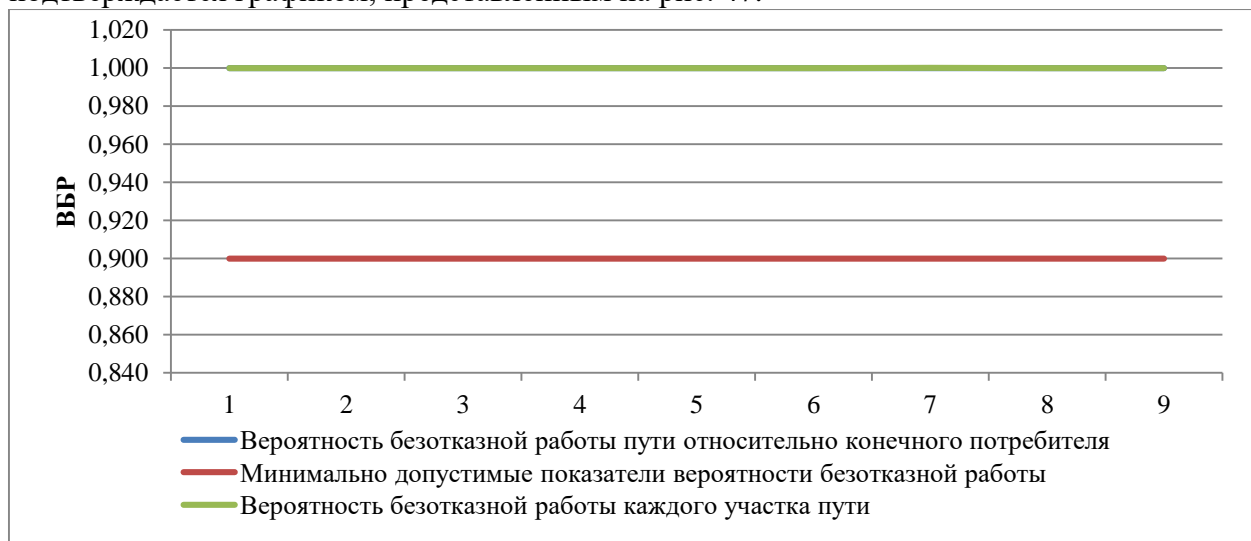
Рисунок 47. ВБР относительно участка тепловой сети от камеры «Вывод - Котельная № 29» до потребителя «Базарная площадь, магазин»
