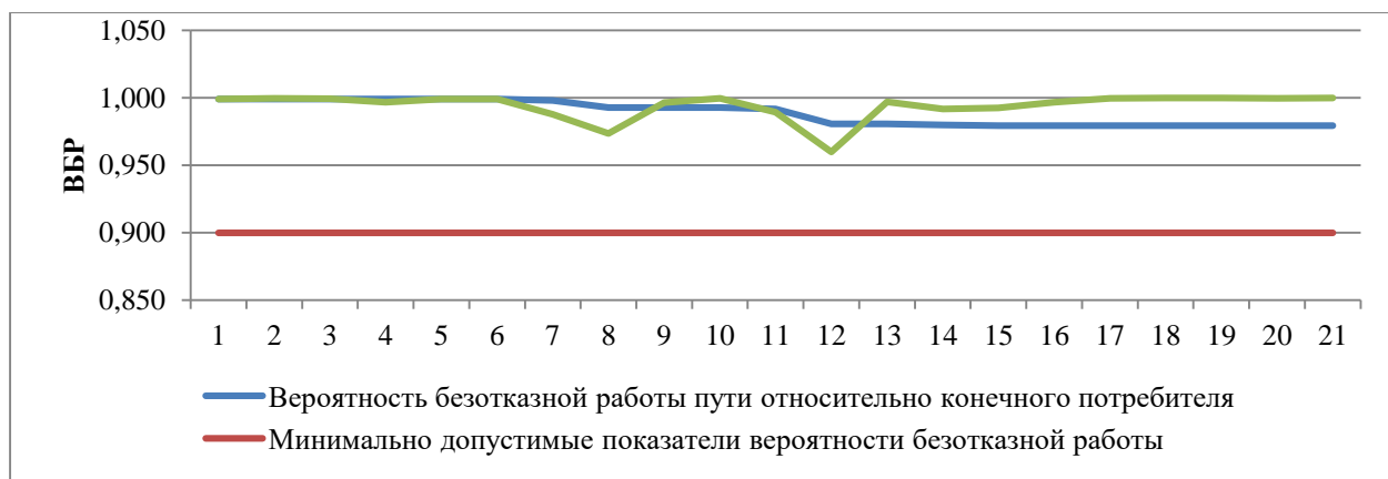
Рисунок 23. ВБР относительно участка тепловой сети от камеры «Котельная № 4» до потребителя «Детский сад № 12»
