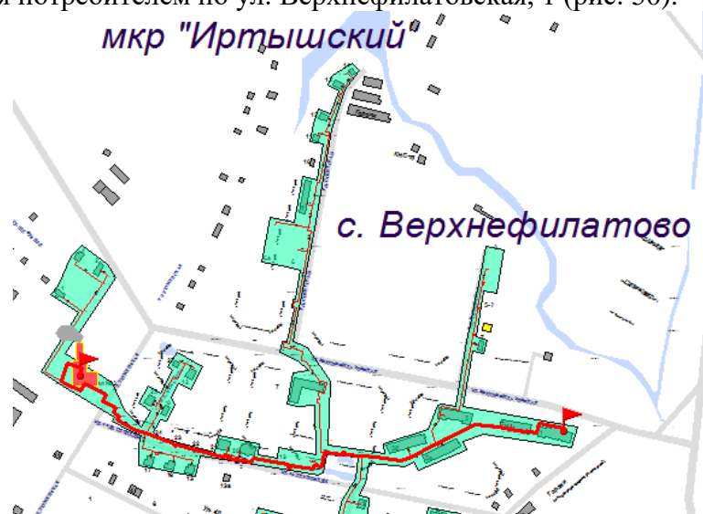
Рисунок 50. Трассировка участка тепловой сети от камеры вывод Котельная № 3 до потребителя по ул. Верхнефилатовская, 1
