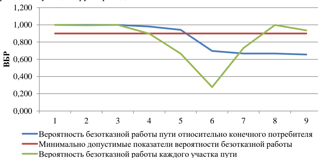
Рисунок 55. ВБР относительно участка тепловой сети от камеры «Вывод - Котельная № 22» до потребителя «Эстетический центр»
