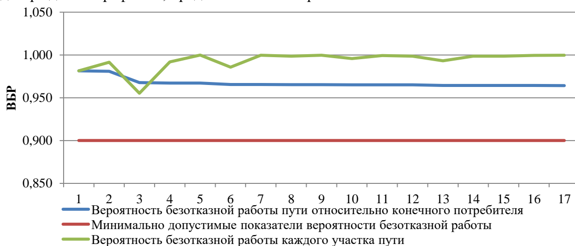
Рисунок 31. ВБР относительно участка тепловой сети от камеры «Вывод - Котельная № 10» до потребителя по ул. Декабристов, 40
