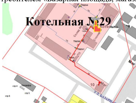
Рисунок 46. Трассировка участка тепловой сети от камеры «Вывод - Котельная № 29» до потребителя «Базарная площадь, магазин»
