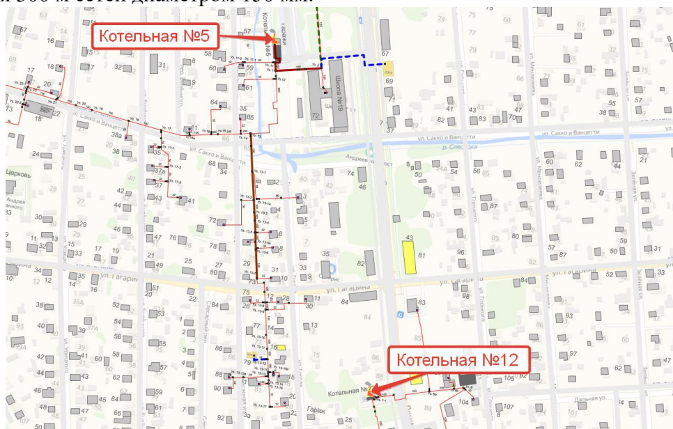
Рисунок 12. Перераспределение нагрузки между котельными № 5 и № 12
