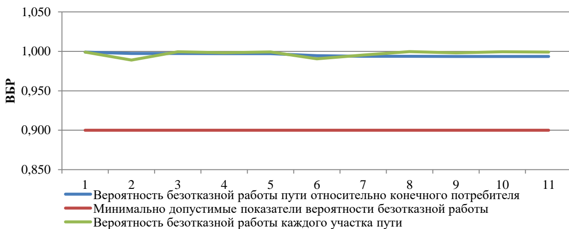
Рисунок 29. ВБР относительно участка тепловой сети от камеры «Вывод - Котельная № 8» до потребителя по ул. Ершова, 2
