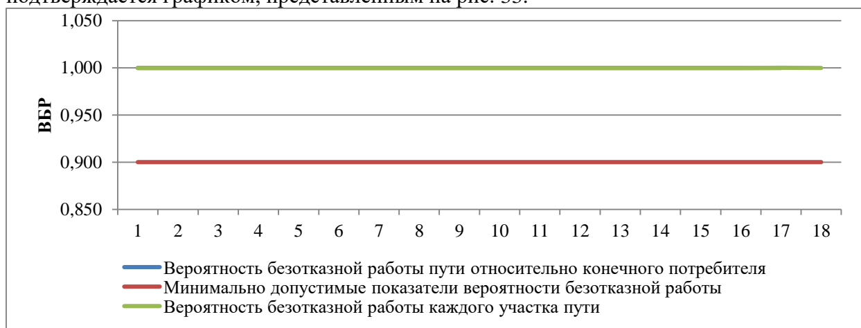
Рисунок 33. ВБР относительно участка тепловой сети от камеры «Вывод - Котельная № 12» до потребителя по ул. Гоголя, 41
