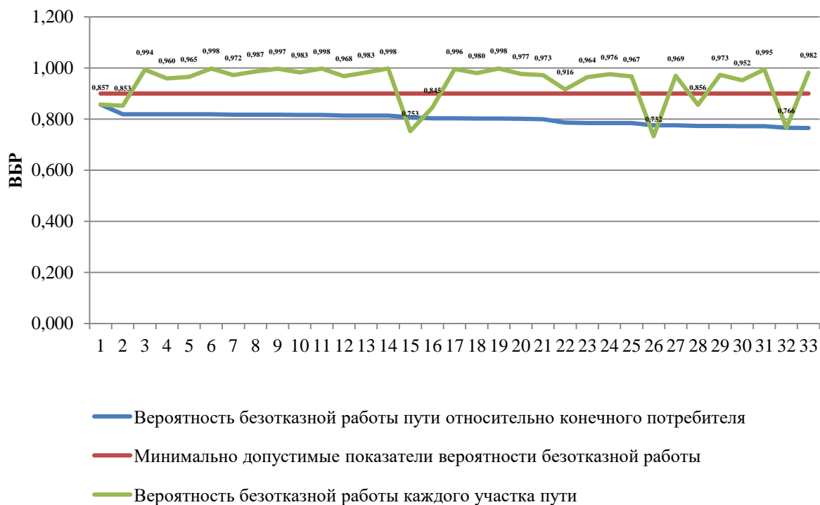
Рисунок 21. Вероятности безотказной работы относительно участка тепловой сети от Тобольской ТЭЦ до Уз. А, Потребитель «Город»
