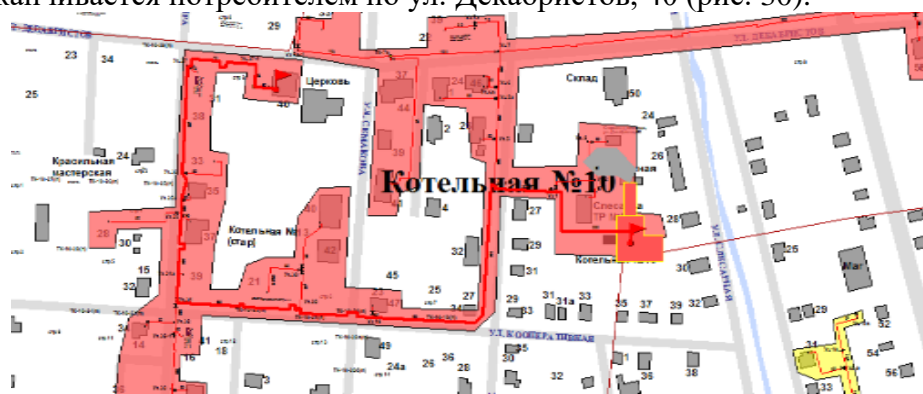
Рисунок 30. Трассировка участка тепловой сети от камеры «Вывод - Котельная № 10» до потребителя по ул. Декабристов, 40
