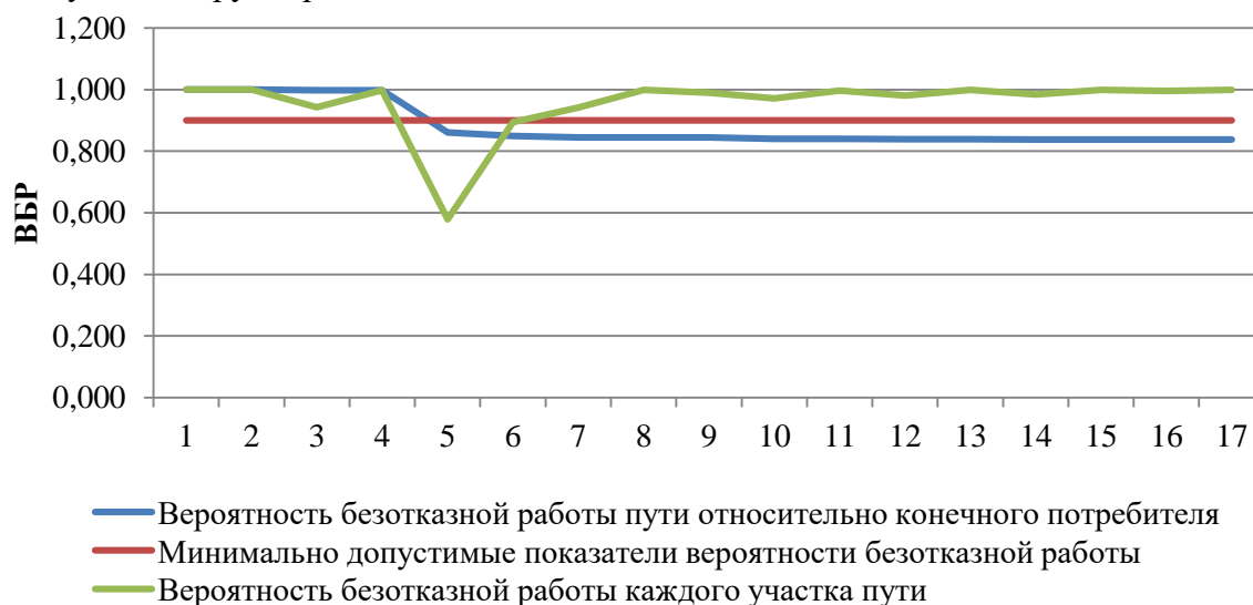
Рисунок 53. ВБР относительно участка тепловой сети от камеры «Вывод - Котельная № 20» до потребителя «Ж/д № 10, КХ «Расчет»
