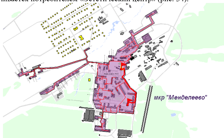
Рисунок 54. Трассировка участка тепловой сети от камеры «Вывод - Котельная № 22» до потребителя «Эстетический центр»
