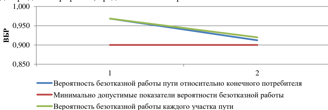
Рисунок 35. ВБР относительно участка тепловой сети от камеры «Вывод -Котельная № 13» до потребителя по ул. 4-я Трудовая, 39
