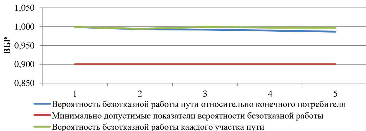
Рисунок 49. ВБР относительно участка тепловой сети от камеры «Вывод - Котельная № 31» до потребителя «Школа № 1, мастерские»
