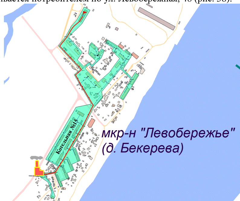
Рисунок 58. Трассировка участка тепловой сети от камеры «Вывод - Котельная № 15» до потребителя по ул. Левобережная, 48
