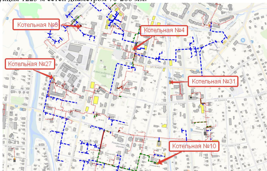
Рисунок 11. Перераспределение нагрузок между котельными №№ 4, 8, 10, 27, 31
