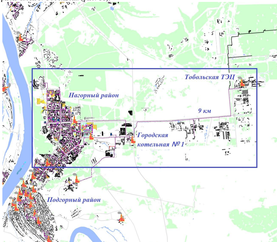
Рисунок 10. Схема размещения источников тепловой энергии для вариантов развития системы теплоснабжения города Тобольска
