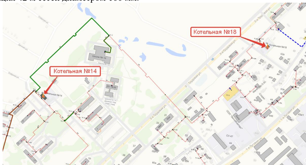
Рисунок 13. Перераспределение нагрузки между котельными № 14 и № 18
