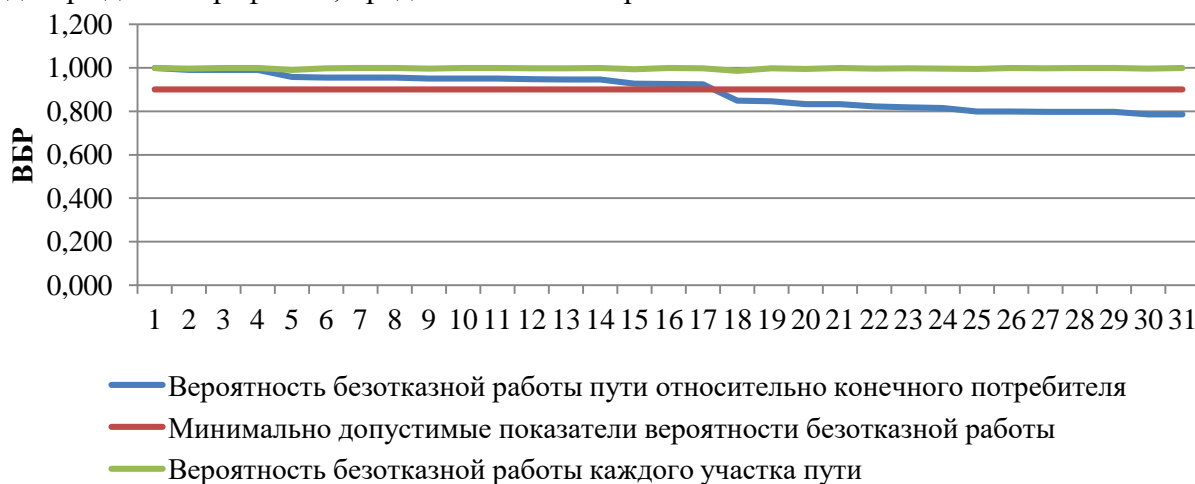
Рисунок 51. ВБР относительно участка тепловой сети от камеры «Вывод - Котельная № 3» до потребителя по ул. Верхнефилатовская, 1
