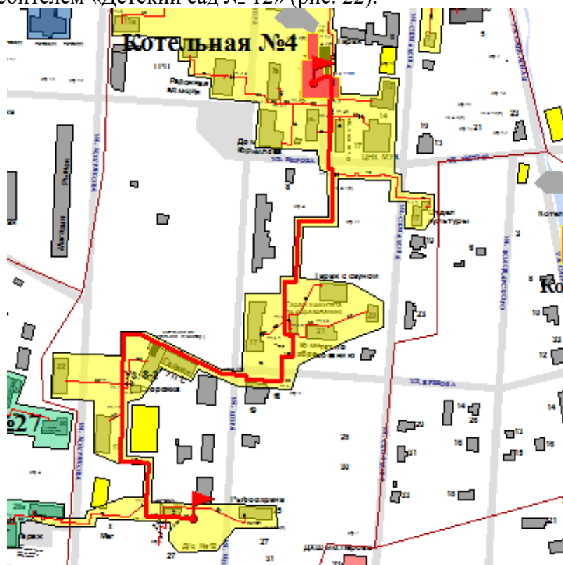
Рисунок 22. Трассировка тепловой сети от камеры «Котельная № 4» до потребителя «Детский сад № 12»
